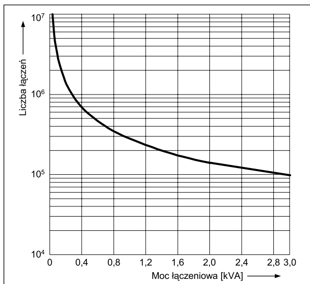
Maksymalna zdolność łączeniowa dla prądu stałego. Obciążenie rezystancyjne Wykres 3
