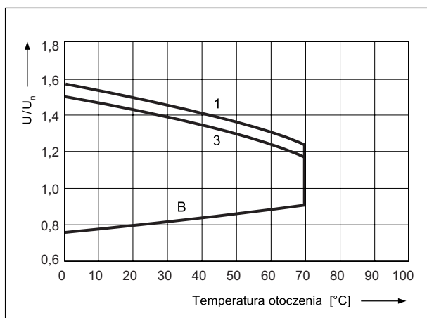
Dopuszczalny zakres napięcia pracy cewki - napięcie przemiennie 50 Hz Wykres 5
