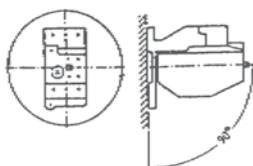
Przełącznik termiczny z adapterem CRI-320 do CRI-350 - do montażu niezależnego
