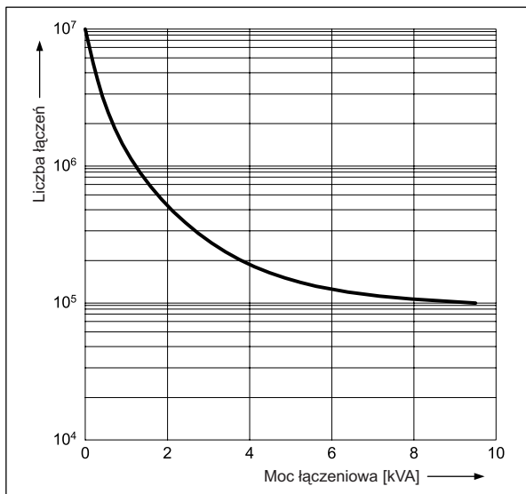
Trwałość łączeniowa w funkcji mocy obciążenia. Obwód bezindukcyjny. Maksymalna częstotliwość łączeń przy obciążeniu znamionowym
